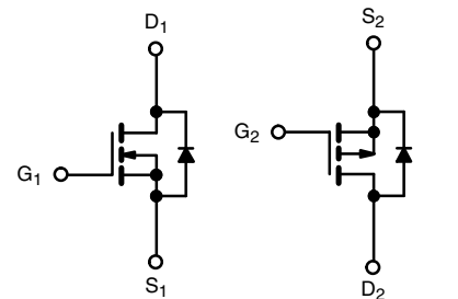
N-Channel MOSFET P-Channel MOSFET
