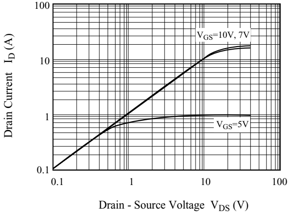
Fig1. I_D - V_{DS}
