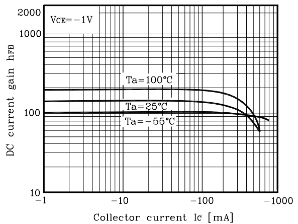
Fig. 6 h_{FE} - I_C
