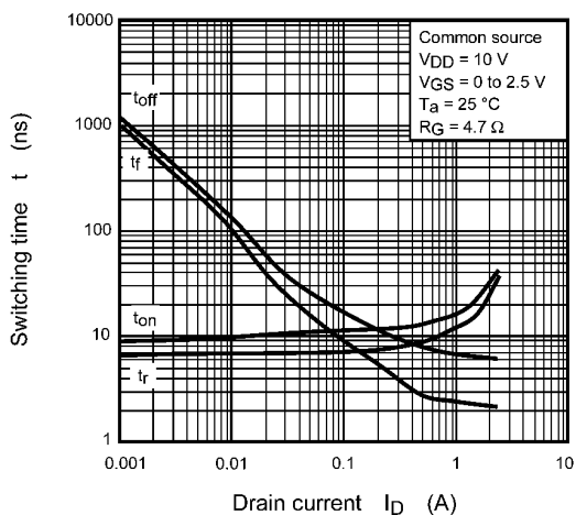
Fig. 7.1.11 t - I_D
