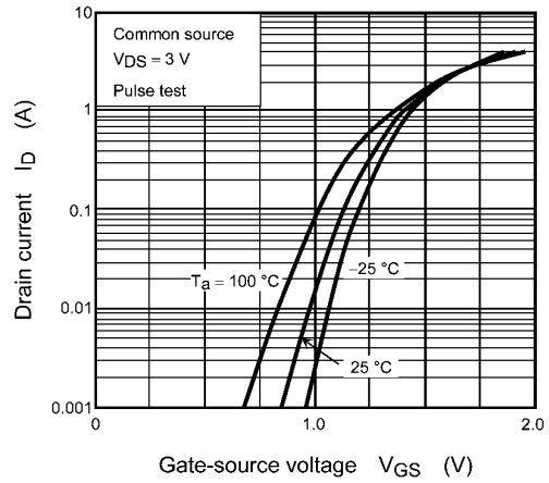
Fig. 7.1.2 ID - VGS
