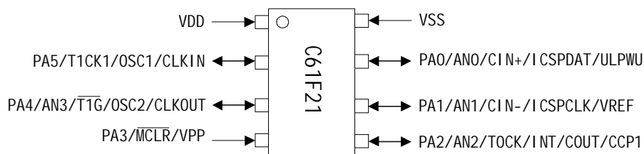
DIP/SOIC/TSSOP 管脚图
