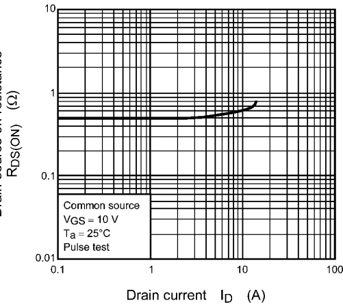
Fig. 8.6 R_{DS(ON)} - I_D
