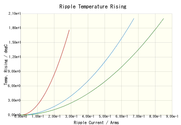
C0603X5R0J224K030BB(100kHz) C0603X5R0J224K030BB(500kHz) C0603X5R0J224K030BB(1MHz)
