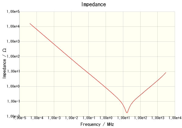
C0603X5R0J224K030BB
