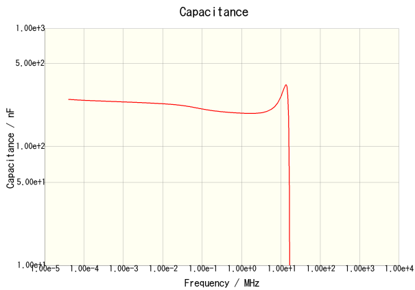
C0603X5R0J224K030BB
