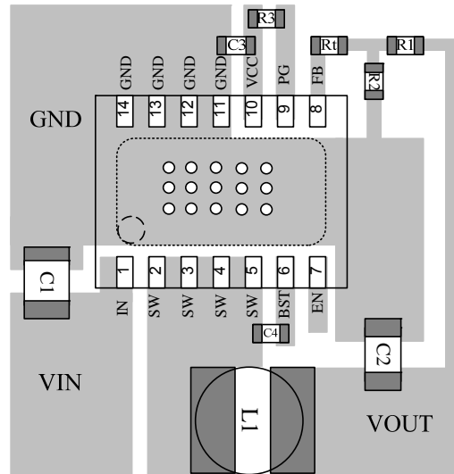
Top Layer
