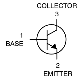
LNST3904F3T5G
