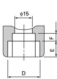
Detail "B" (Conduit conn.)
