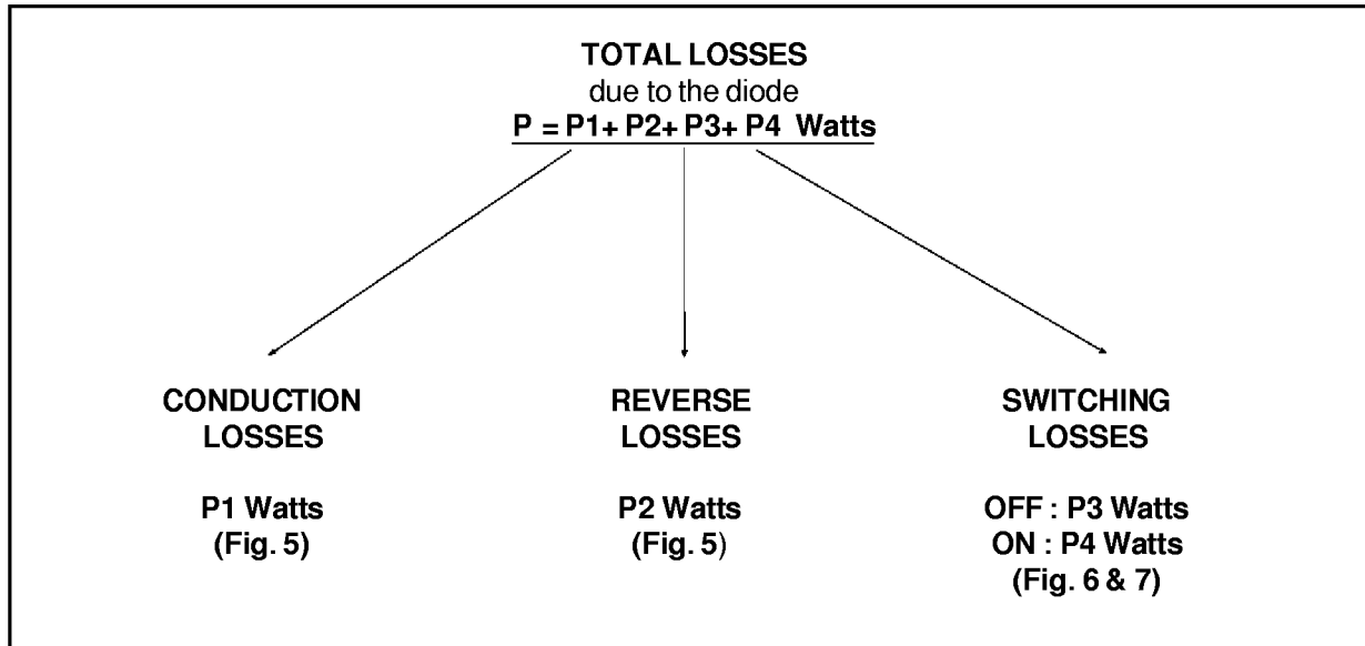
Fig. 1 : SNUBBER DIODE.
