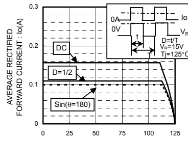
CASE TEMPARATURE : T_c(^{\circ}C) Derating Curve*( I_o - T_c )
