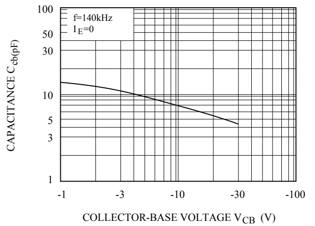
C_{cb} - V_{CB}
