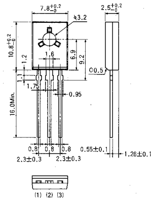
図1 JEDEC: TO-126
