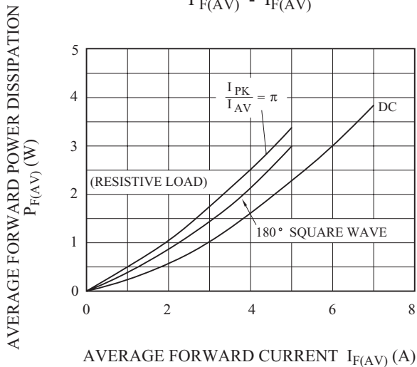
P_{F(AV)} - I_{F(AV)}
