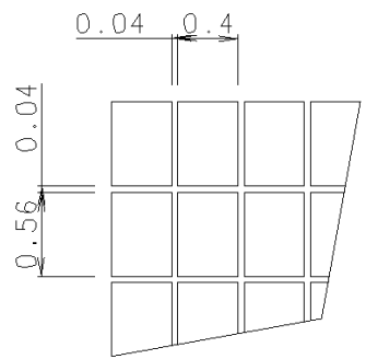
DOT DETALE SCALE 20/1
