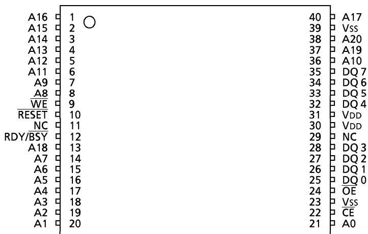
TC58FYT016FT / B016FT (TSOP)
