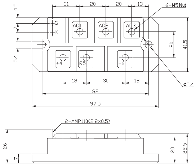
外形寸法図 OUTLINE DRAWING (単位 Dimension : mm)
