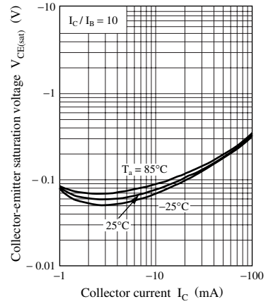
V_{CE(sat)} - I_C
