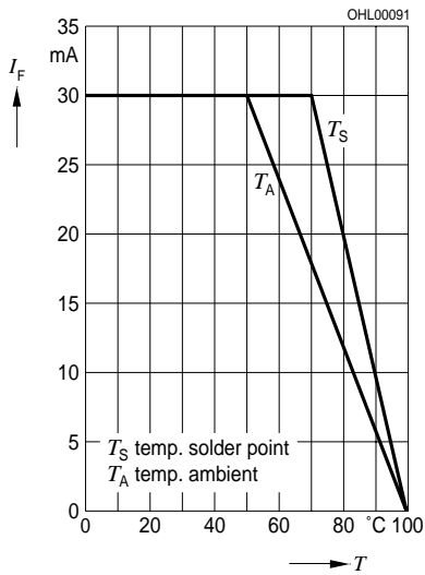
Maximal zulässiger Durchlassstrom I_F = f(T_A) Max. Permissible Forward Current
