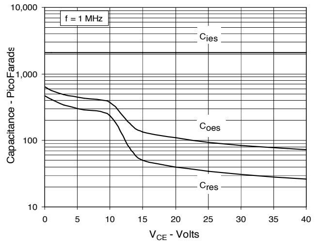
Fig. 16. Capacitance
