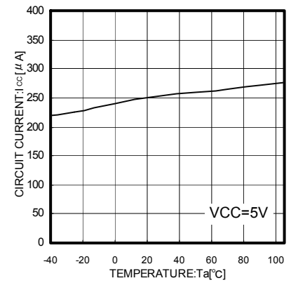
Fig.11 T a - I CC
