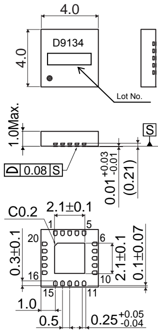
VQFN020V4040(Unit : mm)
