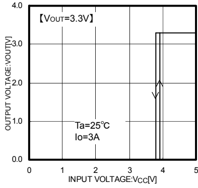
Fig.3 Vcc - VOUT
