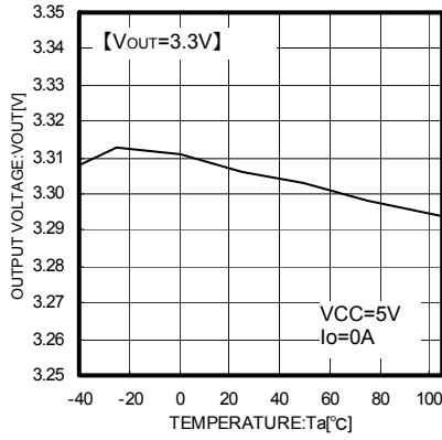
Fig. 6 T a - V OUT
