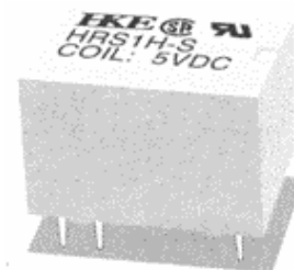
HRS1(H) Relay
