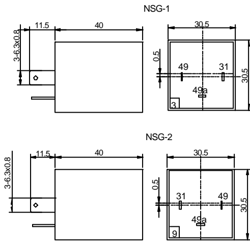
Dimensions
