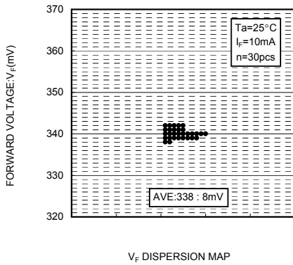
VF DISPERSION MAP
