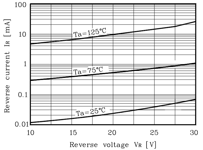
Fig. 2 I_R - V_R
