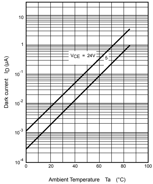
I_D(I_{CEO}) - T_a (typ.)
