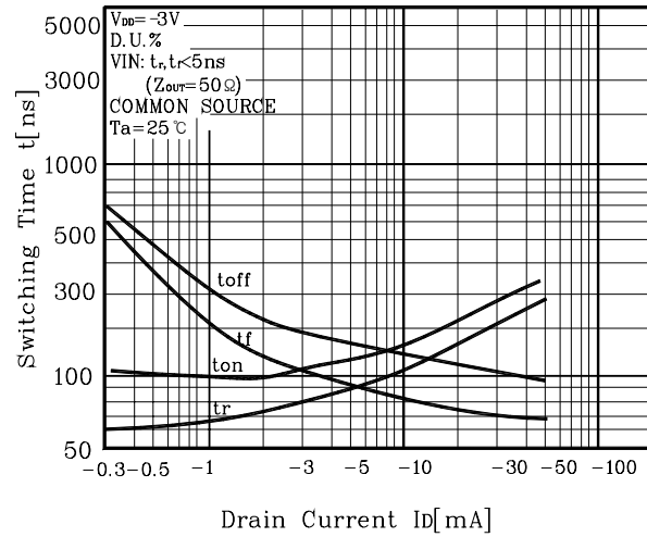
Fig8 t - I_D
