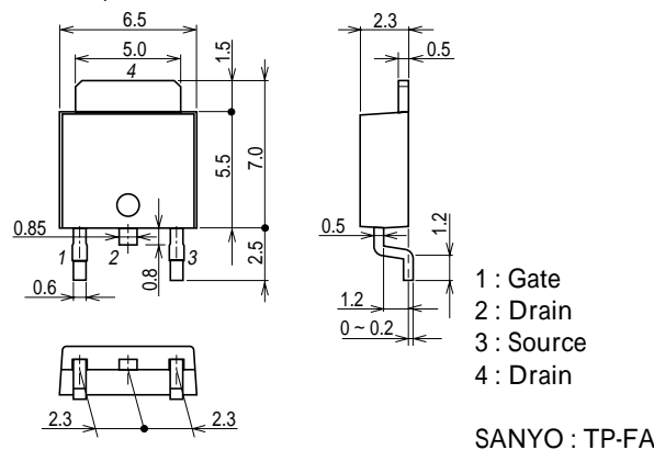
外形図 2092B
