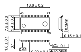
SSOP-B40
