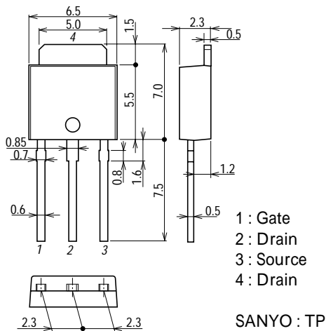
外形図 2083B (unit : mm)
