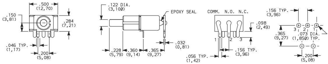
8121SD9RGE SPDT
