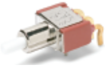
8121SD9A2GE SPDT
