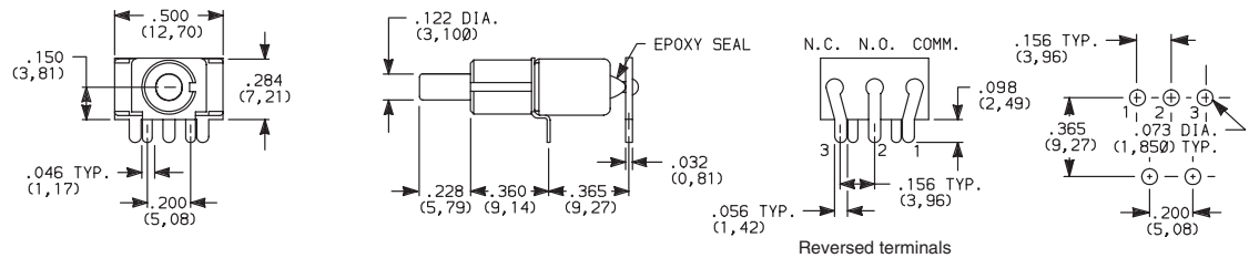
8121SD9R2GE SPDT
