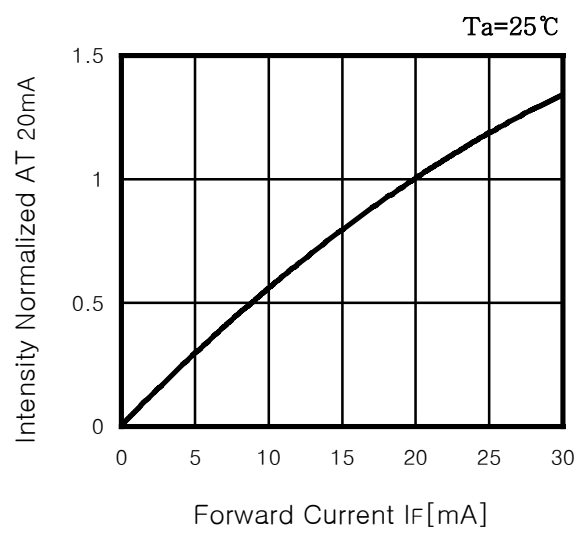
Fig. 2 I_v - I_F
