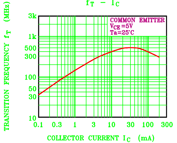
f_T - I_C
