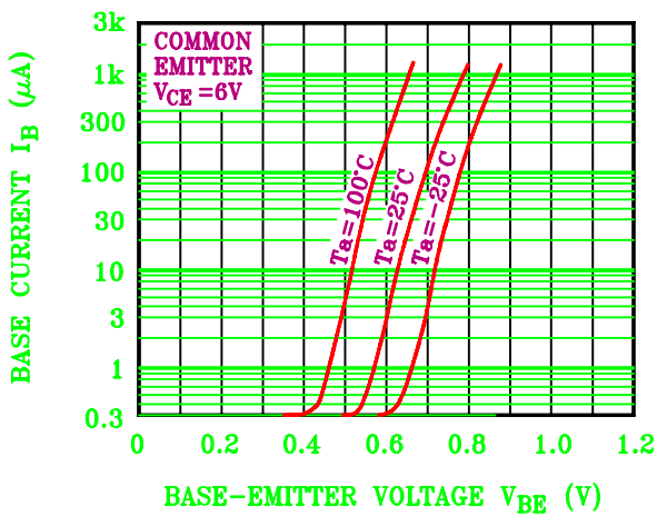
I_B - V_{BE}
