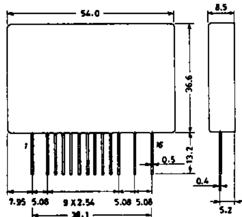
外形図 4059 (unit: mm)
